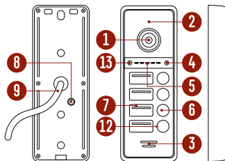
Рис. 7 Вызывная панель FANTASY 4 HD
